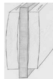
Skisse av langbord med tørkekuv sett fra enden. Margsidene vender utover og kuven gjør at bordene klemmer godt om emnet i øvre, og nedre kant. Illustrasjon: Thor-Aage K. Heiberg.
